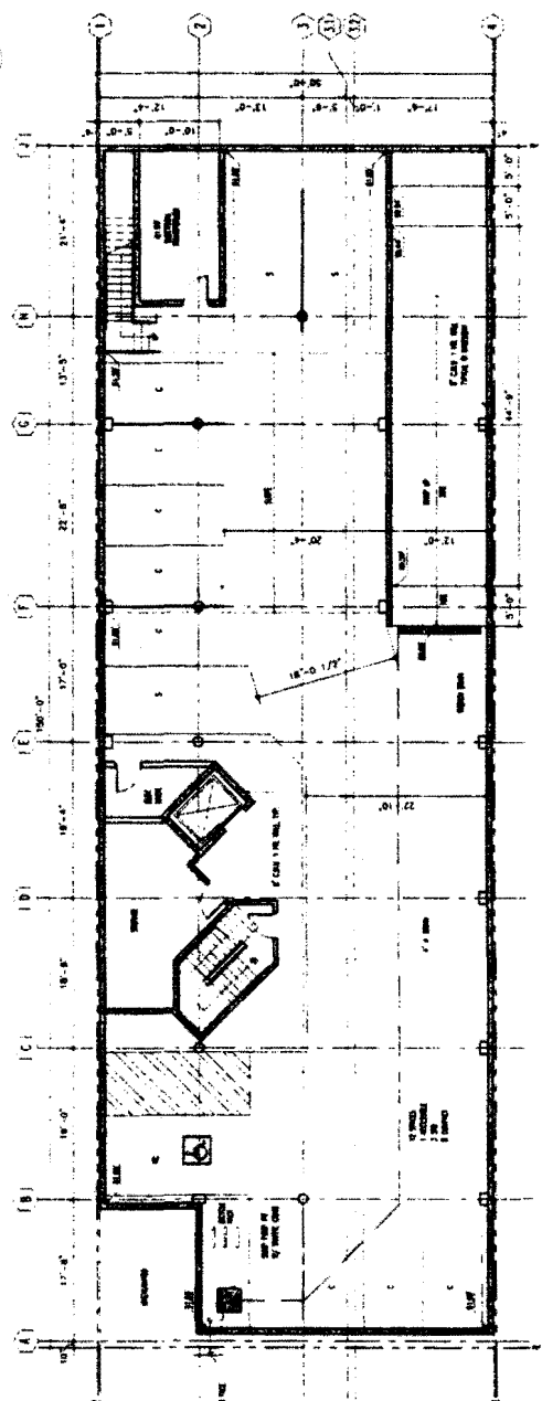
SUBTERRANEAN FLOOR PLAN SCALE: 1/8" = 1'-0"
