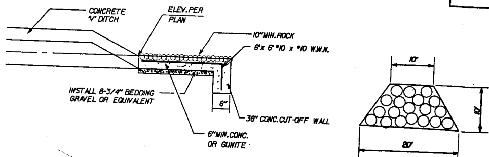
⑥ RIP RAP N.T.S.
