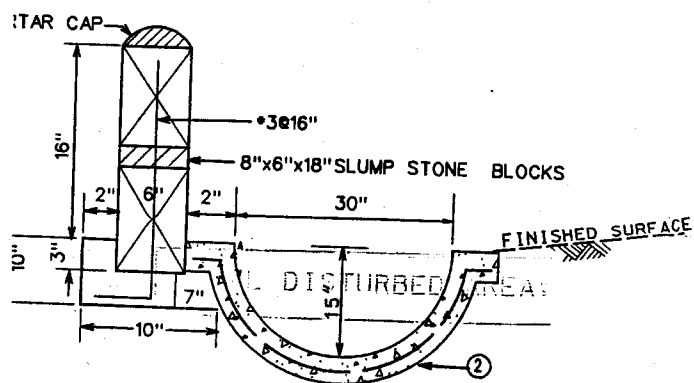
⑤ SPLASH WALL N.T.S.
