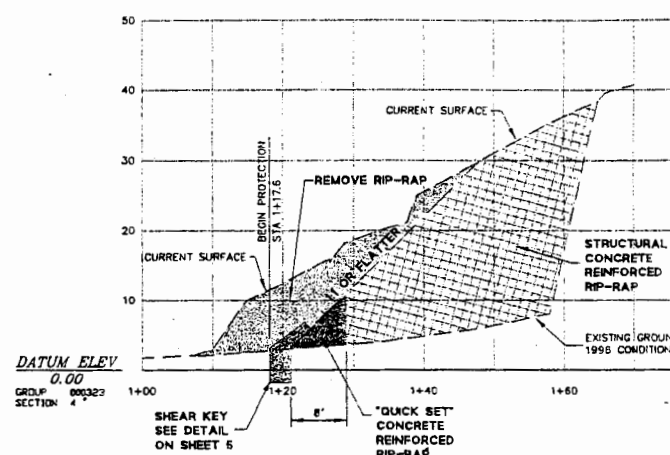
SECTION 4 SCALE: 1"=10' HORIZ & VERT
