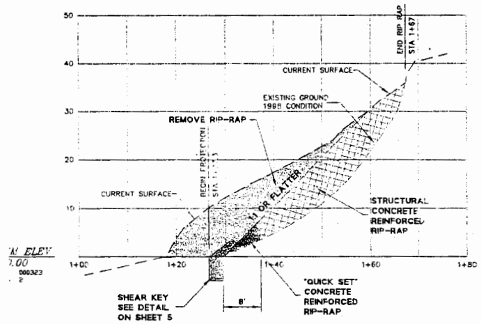
SECTION 2 SCALE: 1"=10' HORIZ & VERT
