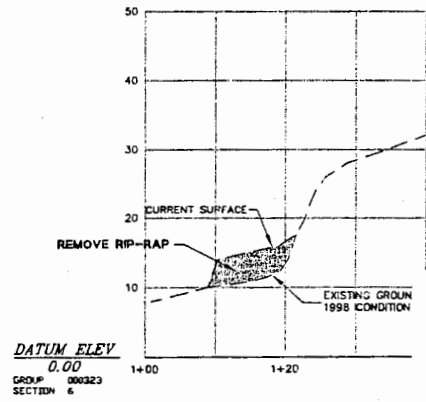
SECTION 6 SCALE: 1"=10' HORIZ & VERT
