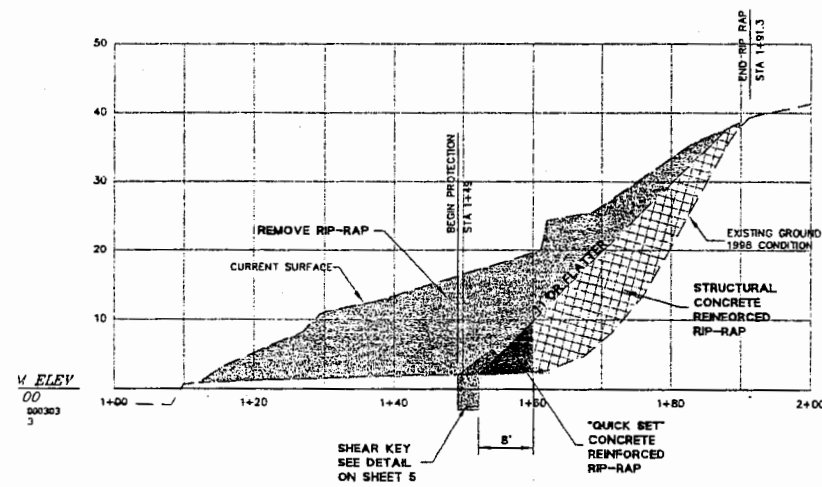
SECTION 3 SCALE: 1"=10' HORIZ & VERT
