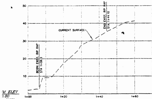
SECTION 1 SCALE: 1"=10' HORIZ & VERT
