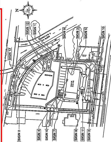
SIGN PLAN SCALE: NONE
